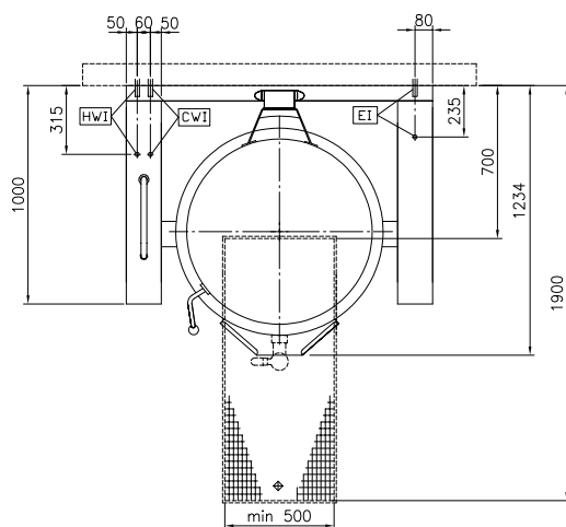
Boven aanzicht
